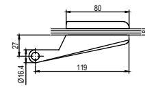
2-teiliges Band SMILE 2-part hinge SMILE
