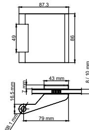
3-teiliges Band SMILE 3-part hinge SMILE
