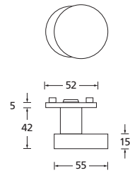
Knopf zyl. versetzt
