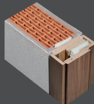
ZARGE F97/PLANO mit gerundeten Kanten in Verbindung mit Plano-Blindstock
