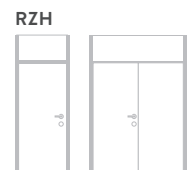
Raumhohe Zarge ohne Querteil mit Kämpfer und Oberlichte bis Raumlichte von 2.600 mm (einflügelig, zweiflügelig)
