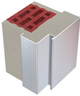
STAHLZARGE PROFIL 42 Umfassungszarge Mauermontage (mitgemauert)
