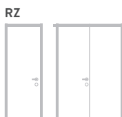
Raumhohe Zarge mit Querteil ohne Kämpfer bis Stocklichhöhe von 2.520 mm (einflügelig, zweiflügelig)
