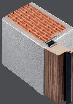
RAHMENSTOCK S-INTERIOR 46 in der Laibung mit Alu-Blindstock montiert
