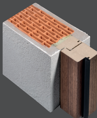
RAHMENSTOCK RST in der Laibung mit Blindstock montiert
